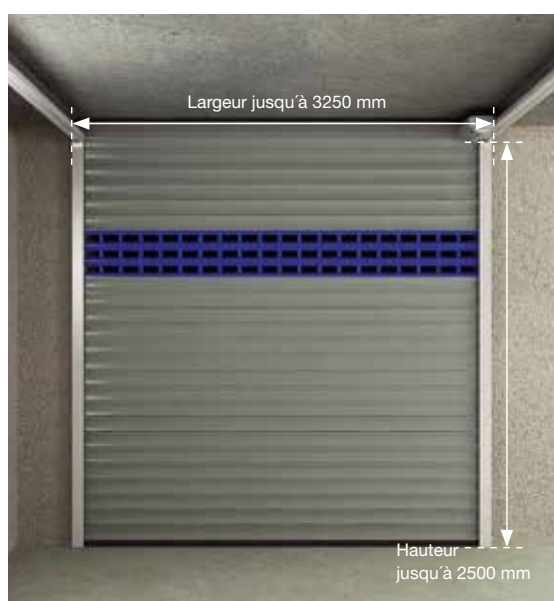
La porte à refoulement plafond GECCO est particulièrement adaptée aux garages individuels disposant de peu de place.
